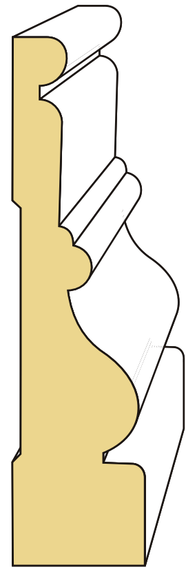
LDF CA4 1" x 4"
