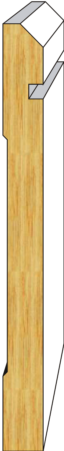
BA 714EPP 11/16" x 7-1/4"
