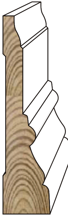
M3 13/16" x 3-3/8"
