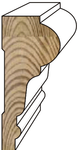
392 1-1/16" x 2-3/8"
