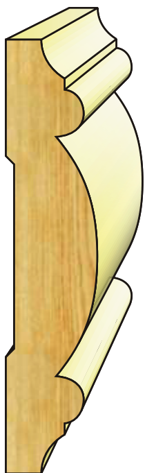
CH 314 11/16" x 3-1/4"
