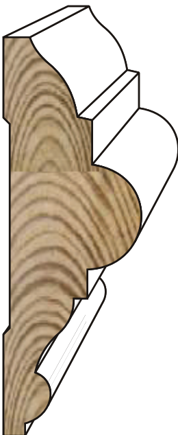
300 1-1/16" x 3"
