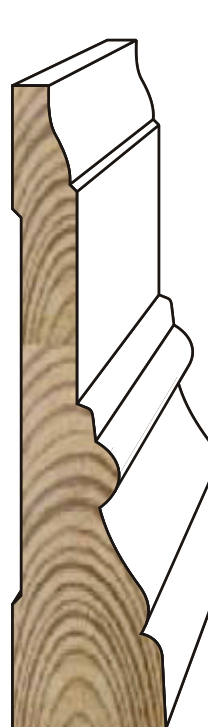
M3 13/16" x 3-3/8"
