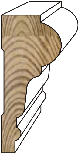
392 1-1/16" x 2-3/8"
