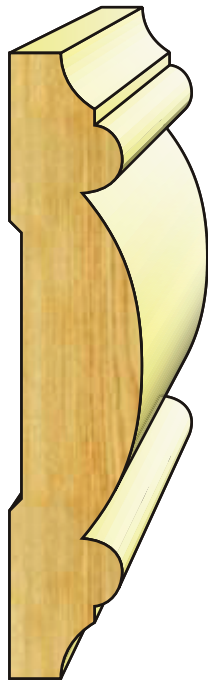
CH 314 11/16" x 3-1/4"
